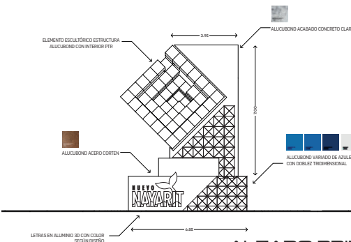
ALZADO PRINCIPAL SIN ESCALA
